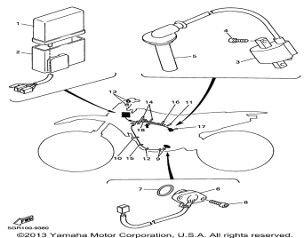
Электрические компоненты 1
