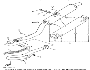
Глушитель
