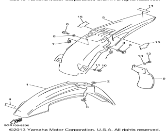
Крыло
