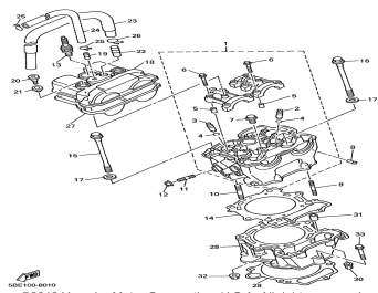
Цилиндр
