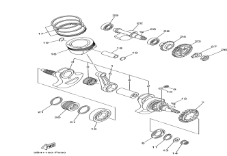
©2014 Yamaha Motor Corporation, U.S.A. All rights reserved. Поршневая группа
