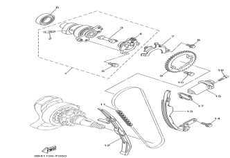
©2014 Yamaha Motor Corporation, U.S.A. All rights reserved. Компоненты ГРМ и распредвал
