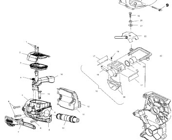
Ручной стартер
