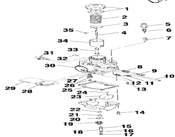
Карбюратор
