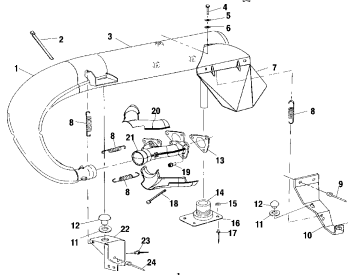
Выхлопная система
