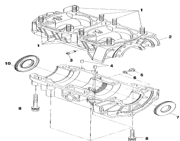
Картер двигателя
