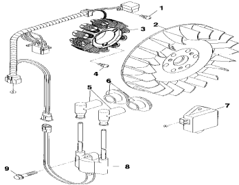
Magneto - s01sd5bs
