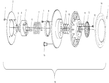
Вариатор
