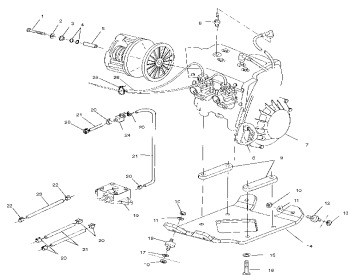
Двигатель и крепления
