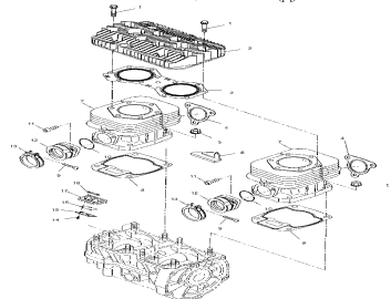
Цилиндр
