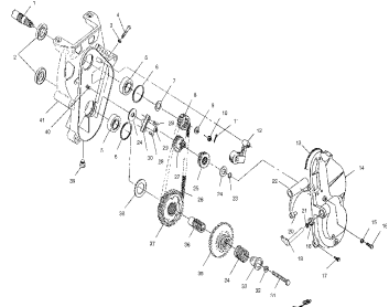
Коробка передач
