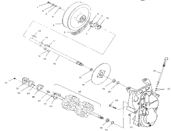
Приводной механизм
