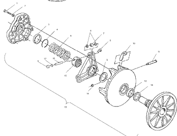
Вариатор
