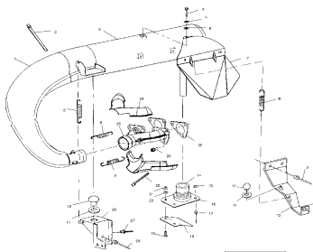
Выхлопная система
