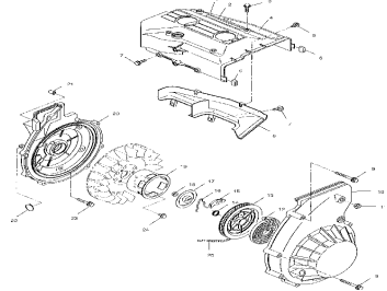
Ручной стартер
