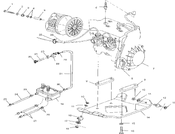
Двигатель и крепления
