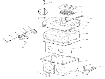
Корпус воздушного фильтра
