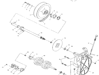
Приводной механизм
