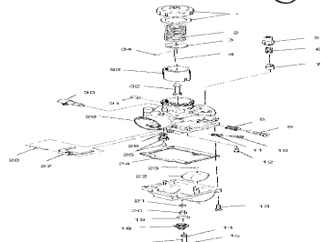
Карбюратор
