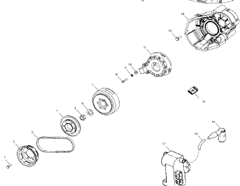
Magneto - e99ss6du
