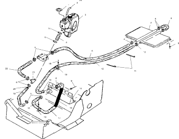
Система охлаждения
