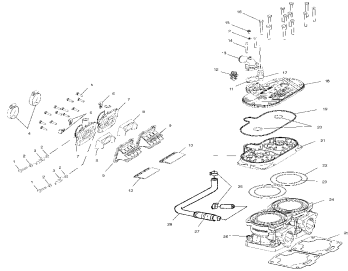
Цилиндр
