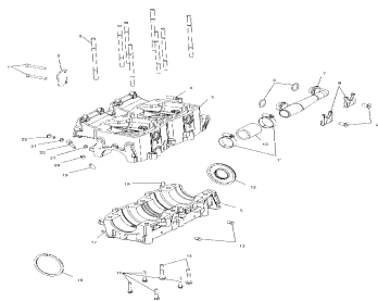
Картер двигателя
