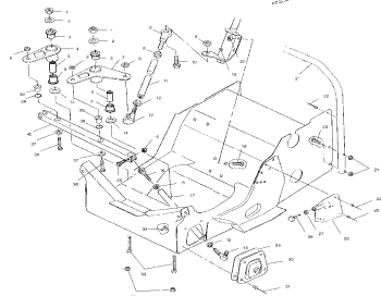
Steering - e99ss6du
