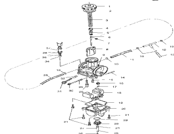
Карбюратор
