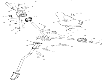
Steering - handlebar - e99ss6du
