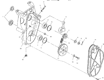
Коробка передач
