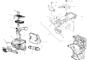
Тормозная система
