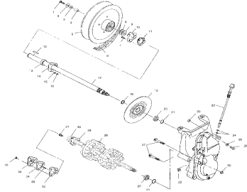
Приводной механизм
