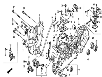
Картер двигателя
