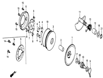
Вариатор
