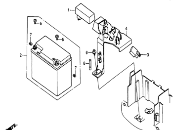
Аккумуляторная батарея
