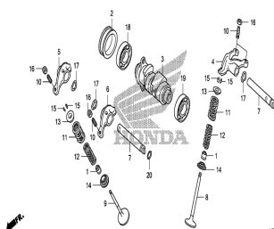
Клапана и распредвал
