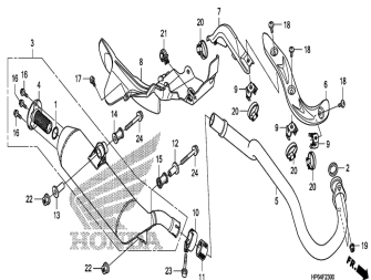
Muffler
