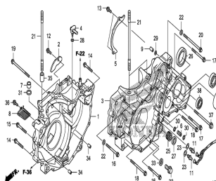
Картер двигателя
