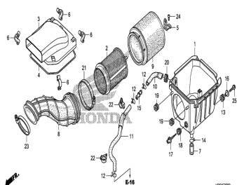
Воздушный фильтр
