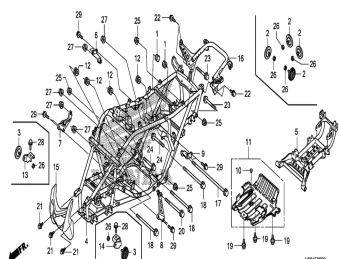
1P961800 Frame
