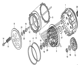
Сцепление
