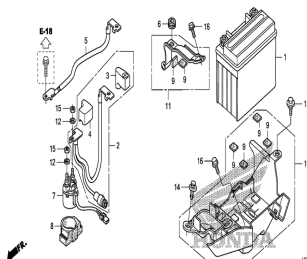
Аккумуляторная батарея
