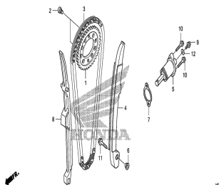
Компоненты ГРМ
