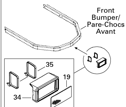
Front Reflector (Europe)/ Réflecteur Avant (Europe)
