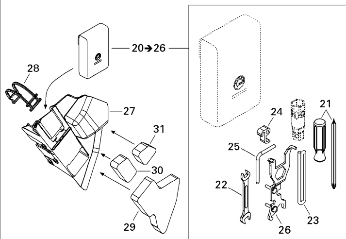
Tool Kit/ Trousse d'Outils
