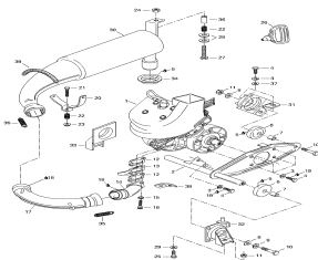
Двигатель и глушитель
