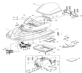
Капот и стекло
