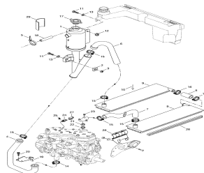
Система охлаждения
