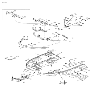
Воздухозаборник
