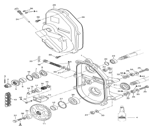
Коробка передач
