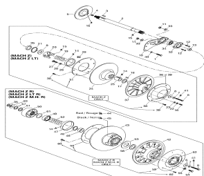
Шкив вариатора
