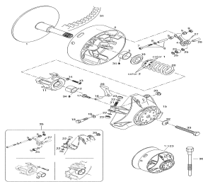
Вариатор
