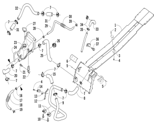
Система охлаждения
