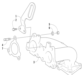
Выпускной коллектор
