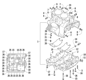
Картер двигателя
