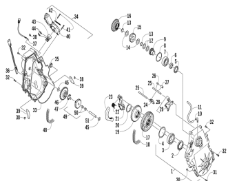
Корпус трансмиссии
