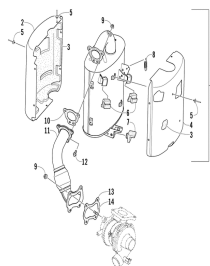
Глушитель
