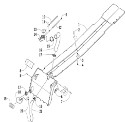
Система охлаждения
