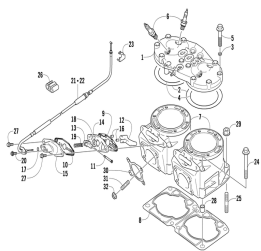
Головка блока цилиндров и цилиндр
