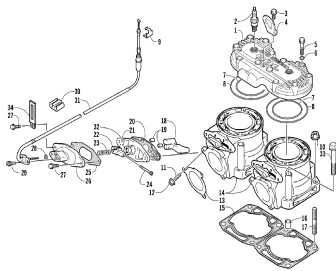
Головка блока цилиндров и цилиндр
