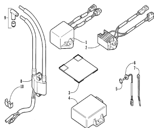
Электрические компоненты
