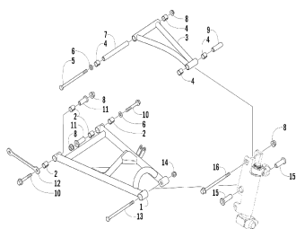
Рычаги подвески
