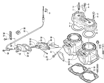
Головка блока цилиндров и цилиндр
