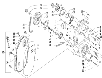
Детали трансмиссии
